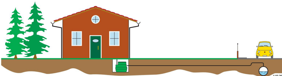
Asennusesimerkki
